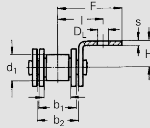
A2 einseitige Winkelaschen bent attachments, one side
