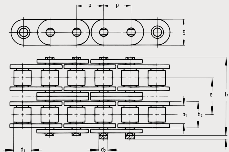
Verschlussseite / Connecting side
